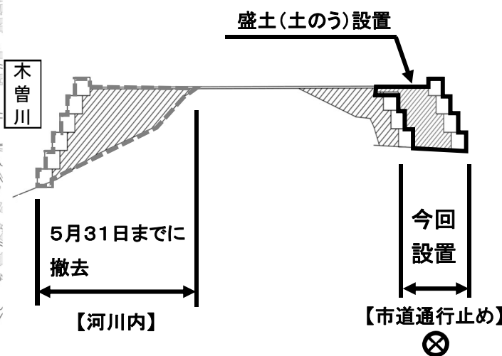
A-A 断面図
