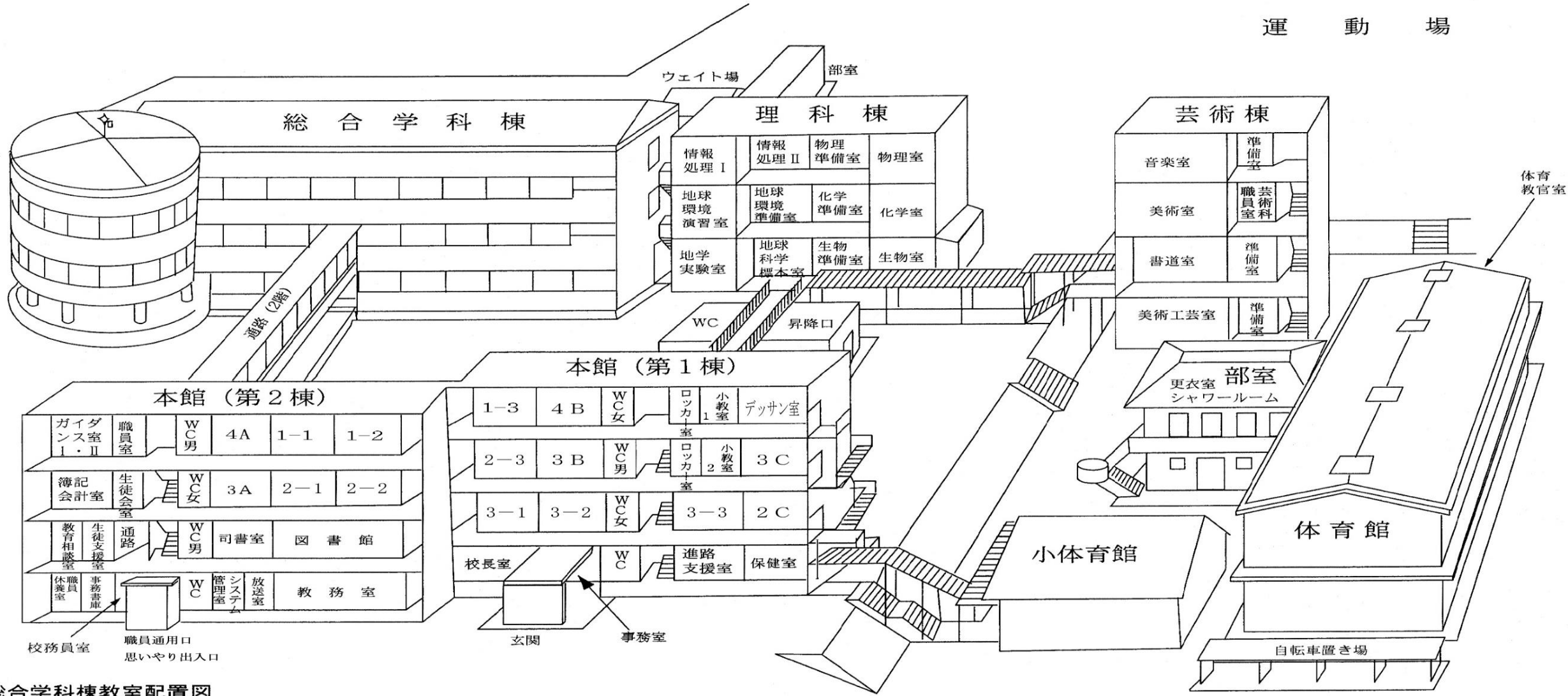
総合学科棟教室配置図
