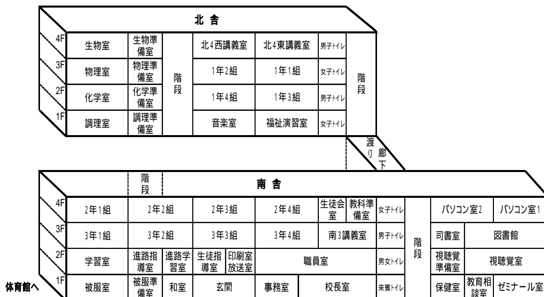
教室配置図
