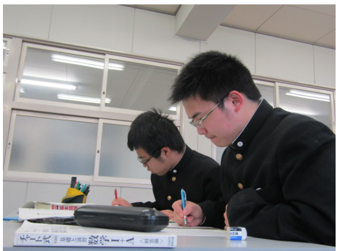
数学
