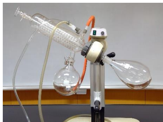
図7 減圧蒸留装置
