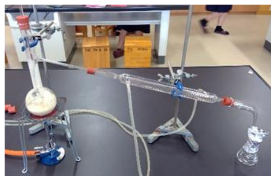
図6 常圧蒸留装置
