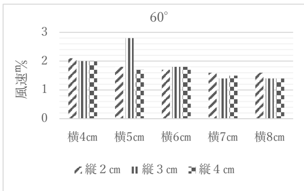
図10 角度 60° での風速 (m/s)
