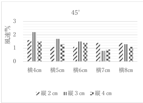
図9 角度 45° での風速 (m/s)
